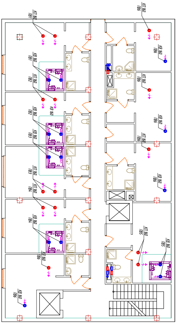
Вентиляция. План 4-20 этажа.
